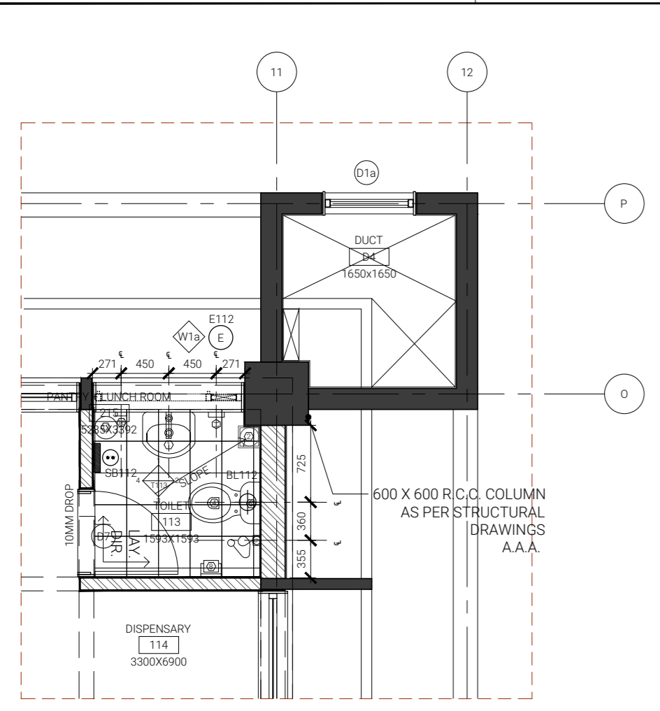
1 PLAN 1:50
