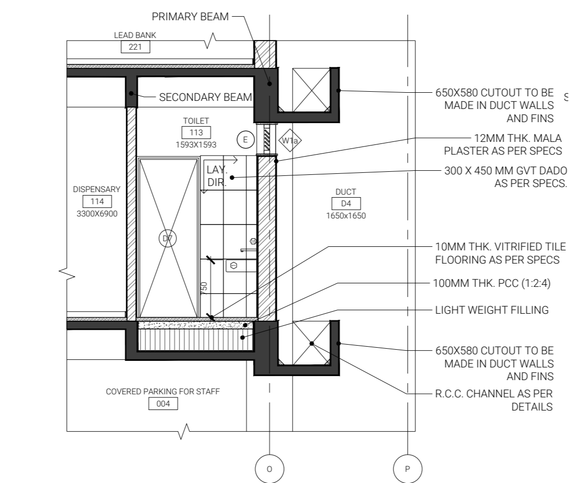
2 ELEVATION 4 1:50
