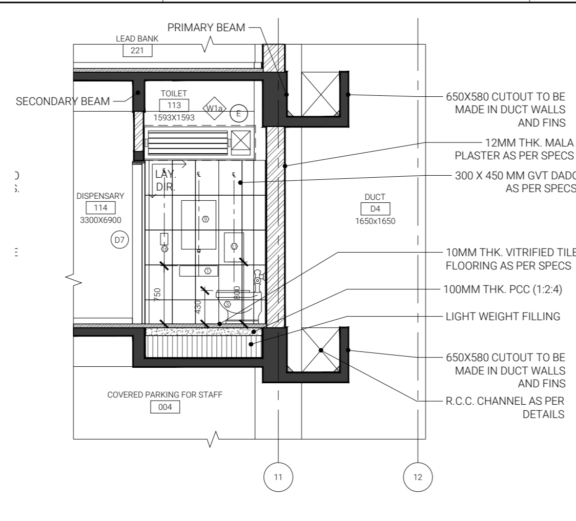
2 ELEVATION 1 1:50
